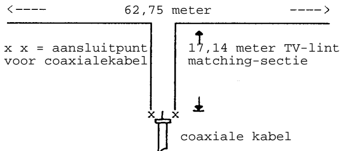
fig. 1 De allband dipool van PAOGHS
