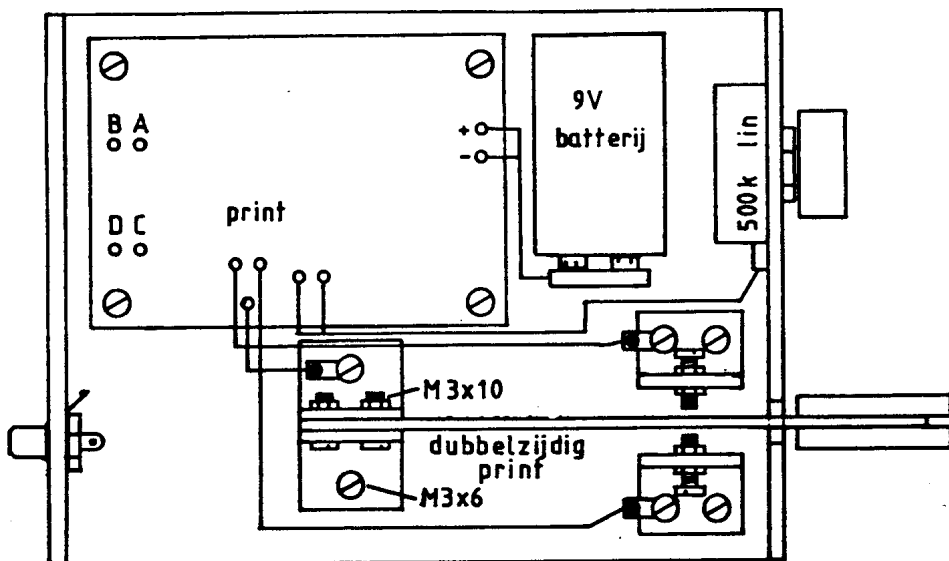
bovenaanzicht
